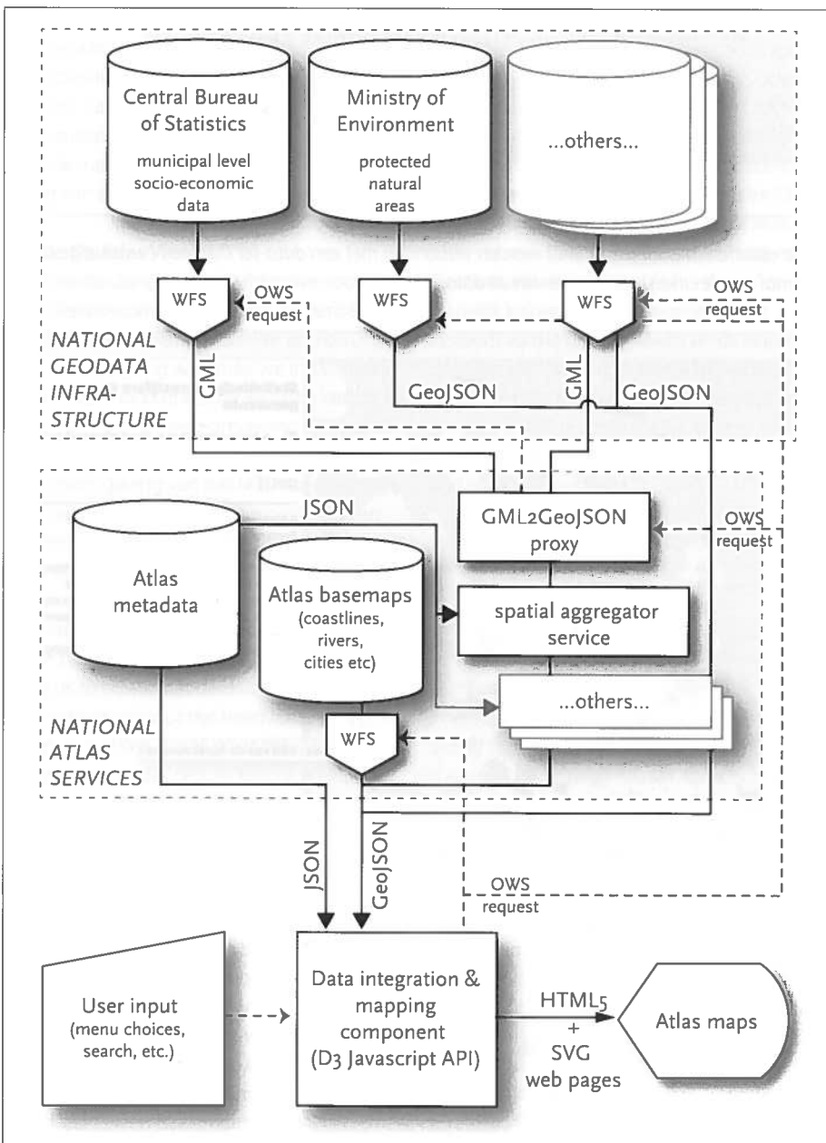
Figuur 2 - Voorgestelde architectuur, een combinatie van de SDI omgeving van het NGDI (boven) met Nationale Atlas services (midden) en de Nationale Atlas kaartviewer voor het Open Web Platform (onder).
